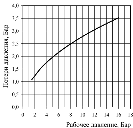
Ду 50 мм
