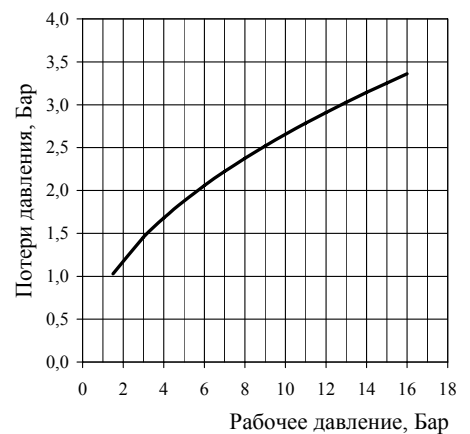
Ду 80 мм
