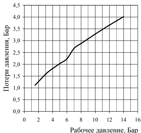
Ду 100 мм
