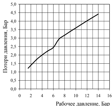
Ду 150 мм
