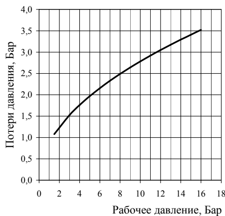
Ду 65 мм
